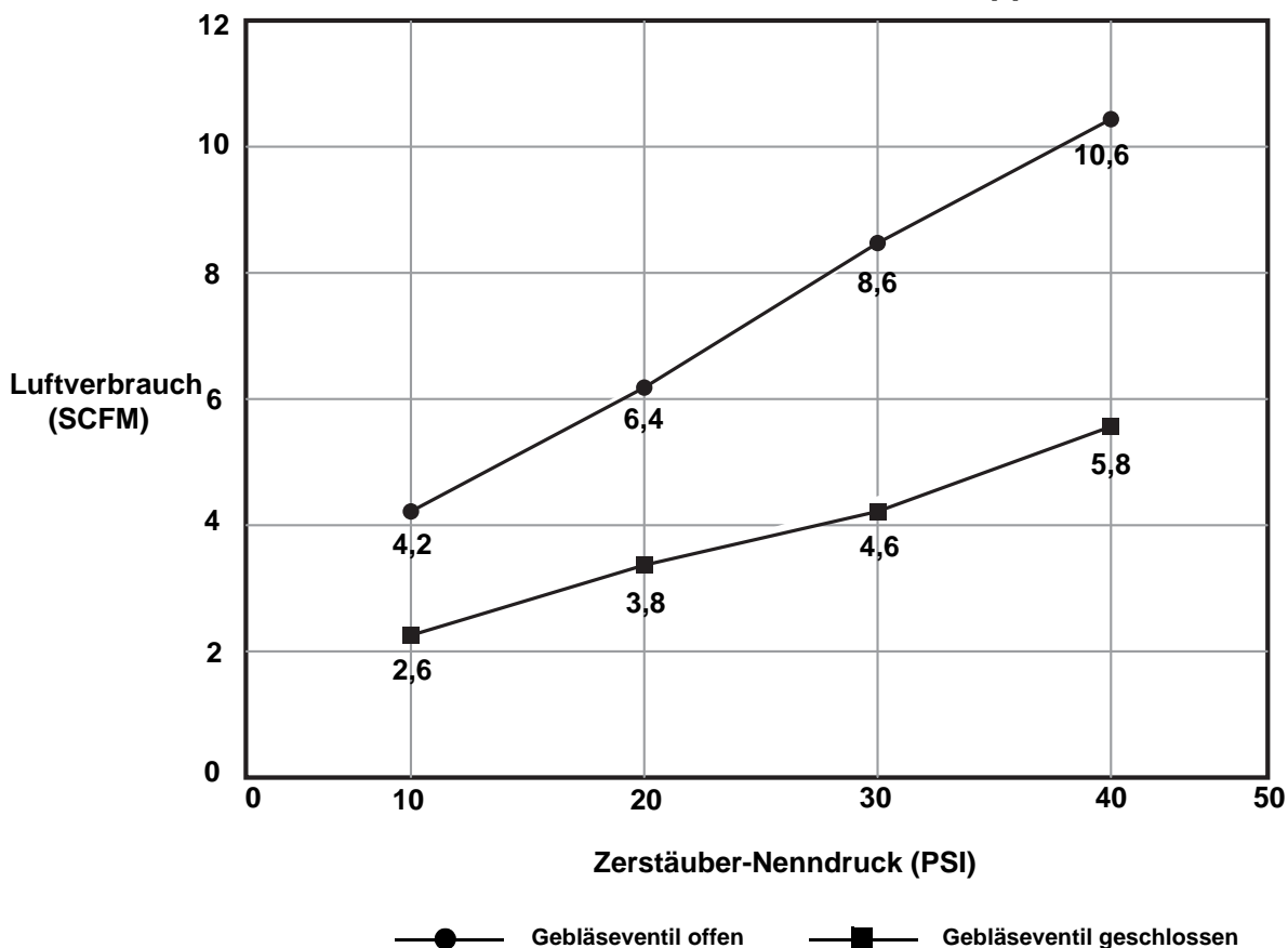
Luftdurchfluß; Standard-Luftkappe
