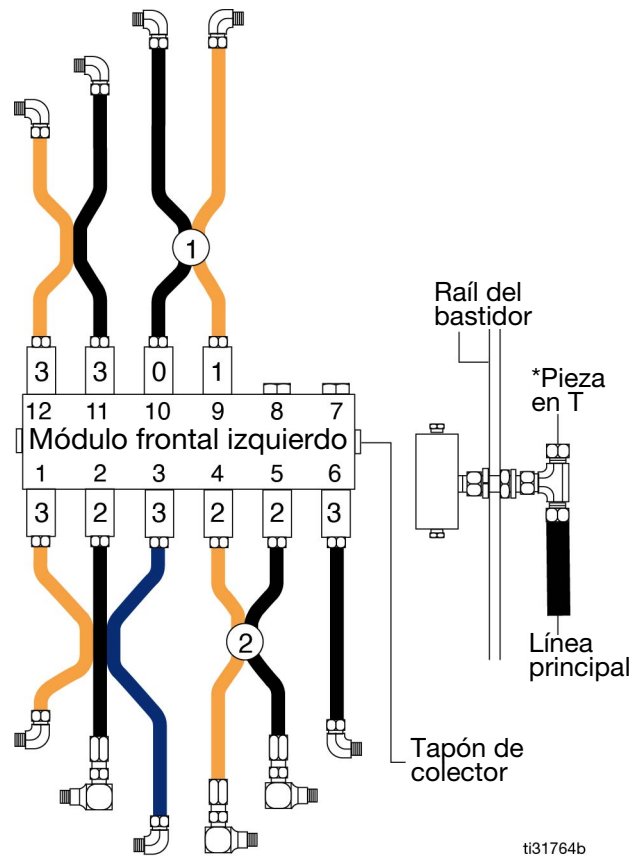
FIG. 49: *Se muestra la pieza en T 129759. También puede usar el codo 129755
