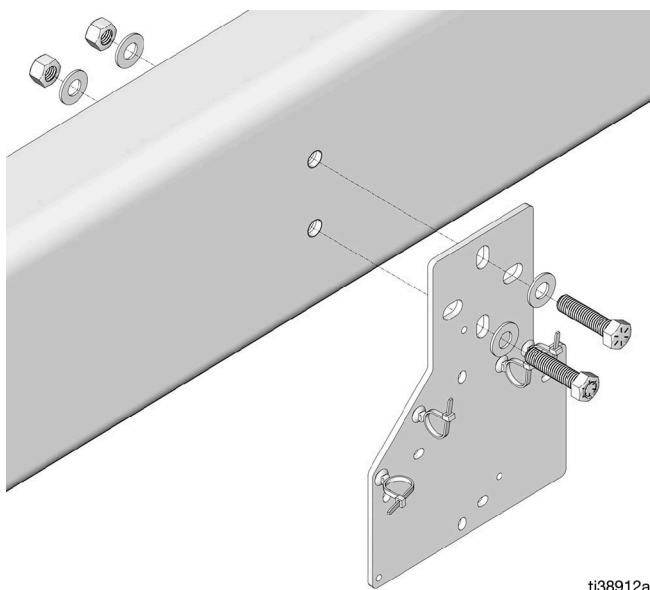
FIG. 11: Montaje de fijación en el exterior del bastidor del camión (Kit 25T767)
